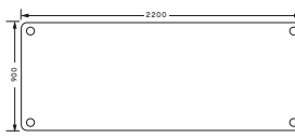
1434 Besprechungstisch 2200x900x750mm 1441 Besprechungstisch 2000x800x750mm 1442 Besprechungstisch 2000x1000x750mm
