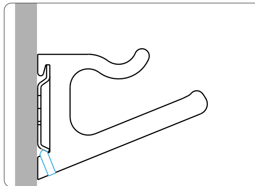
7 Aushängesicherung: Schrauben anziehen! Hanging device safety feature: Tighten the screws!
